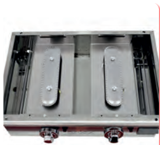
Quemadores ARILEX ARILEX Burners Brûleurs ARILEX
